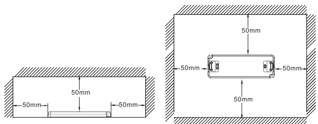
Sugerowany sposób montażu oraz przestrzeń wokół zasilacza
